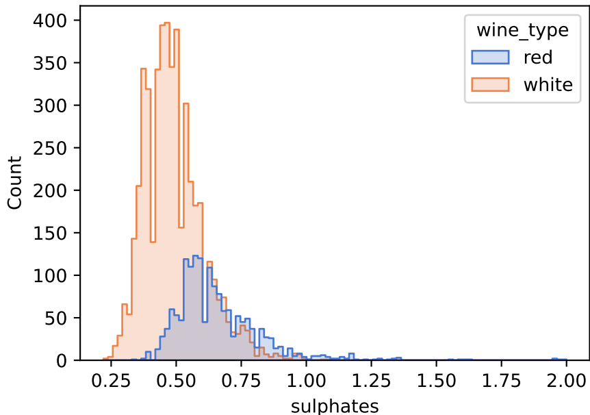
Histograma Incondicional (Bimodalidade) - sulphates
